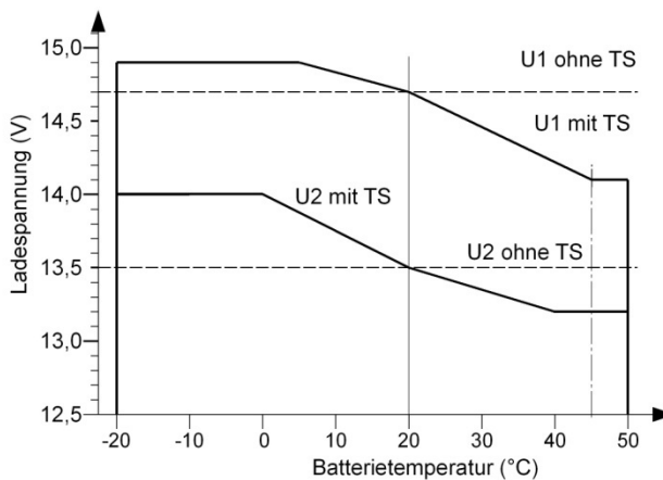
Ladeprogramm „MOTOR“ (FNFV), Kennlinie IU1oU2
